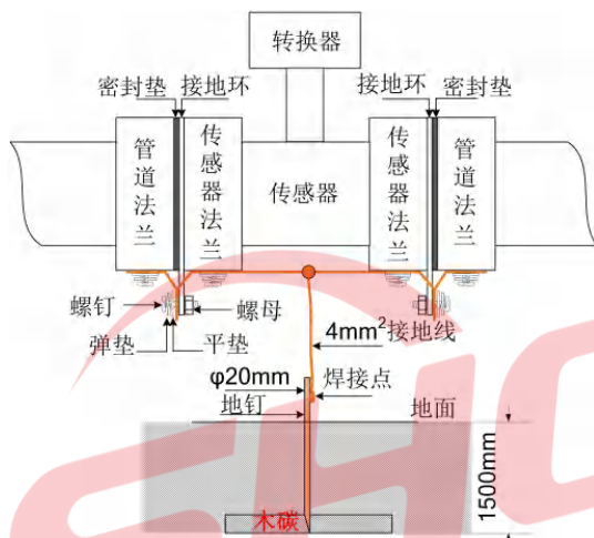
图 1.7 转换器接地示意图
