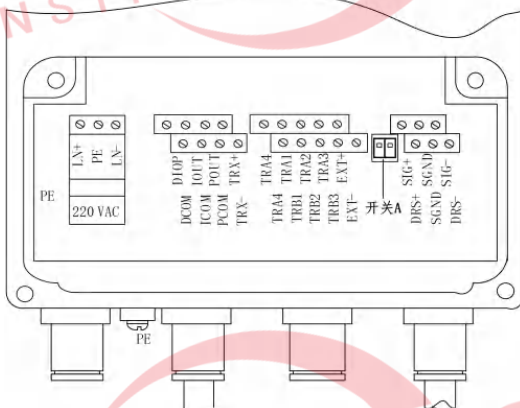
图 1.3 M8RBF22 主板接线端子图
