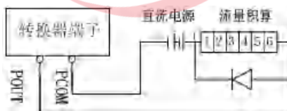
图 1.3 外供电电源接电子计数器
