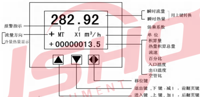
图 3.1 键盘定义与液晶显示
