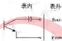
图 1.6 表内 OC 门连接方式
