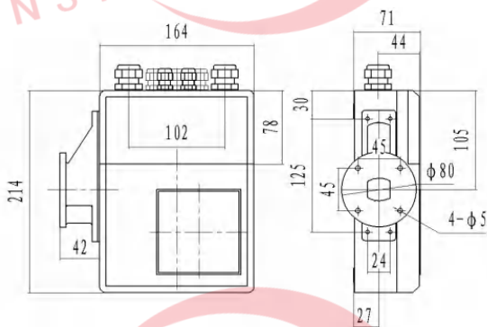
图 4.1 方型壳体分体式外型尺寸图
