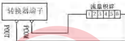
图 1.4 内供电电源接电子计数器
