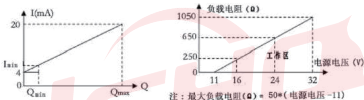
4 ~ 20mA 电流输出特性
