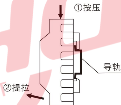
拆卸图
