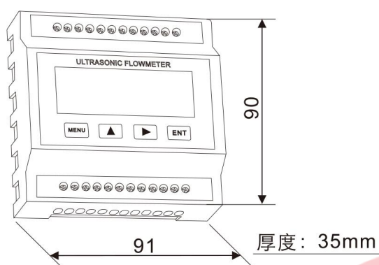
安装图
