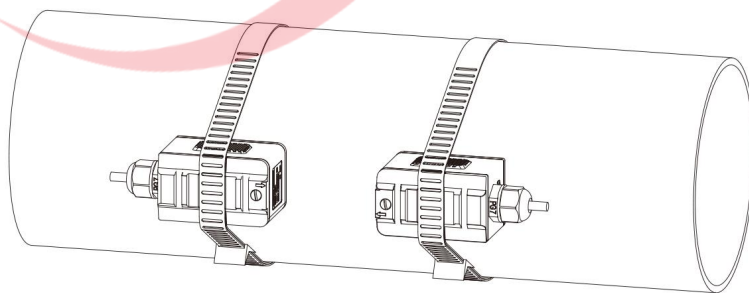
钢带固定 DN15-500
