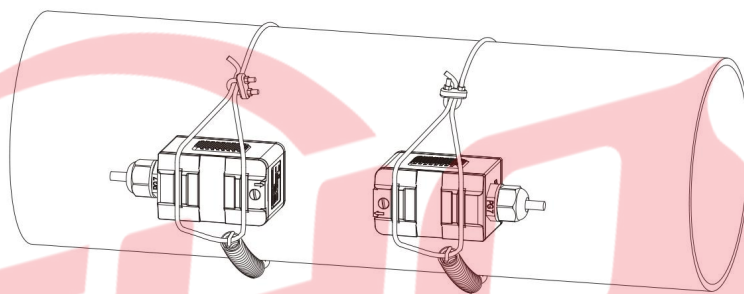
钢丝绳固定 >DN500
