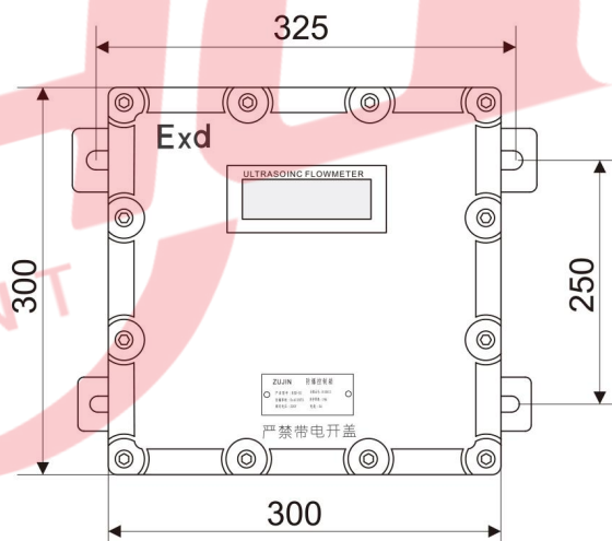
厚度：165mm
