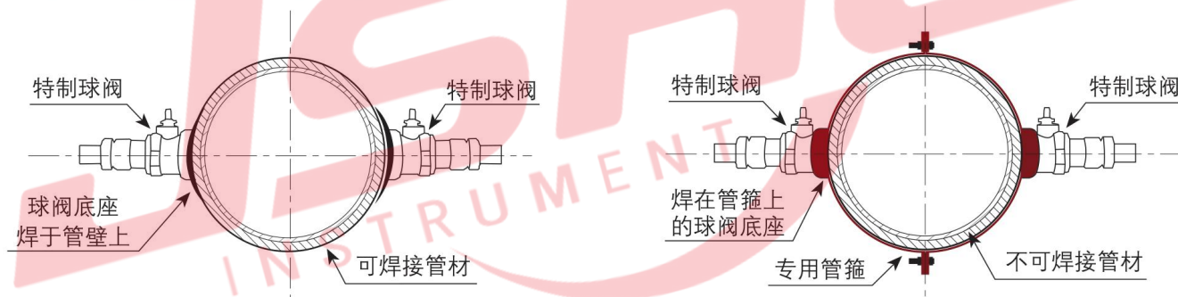
焊接固定球阀底座
