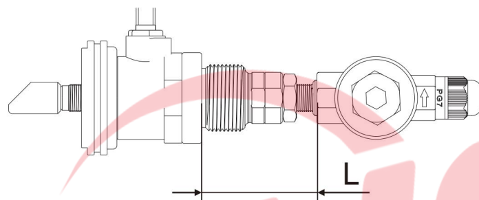
标准插入型传感器安装完成后探头杆留在管道外侧的长度 L=73\text{mm}-\text{壁厚} 加长插入型传感器安装完成后探头杆留在管道外侧的长度 L=202\text{mm}-\text{壁厚} 插入深度安装计算图
