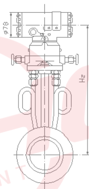
图 4 测蒸汽型
