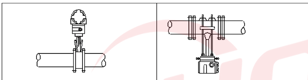
图 7 测蒸汽（夹装式）
