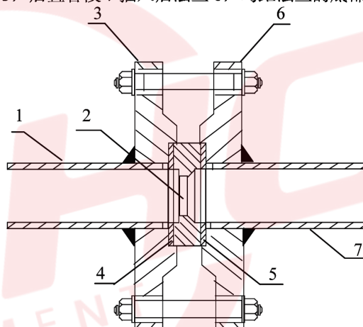
图 13 一体孔板与管道的安装
