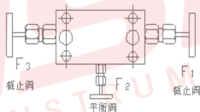
图 1 三阀组结构示意图
