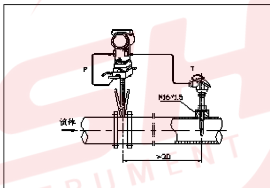
图 12 一体式孔板流量计安装方式
