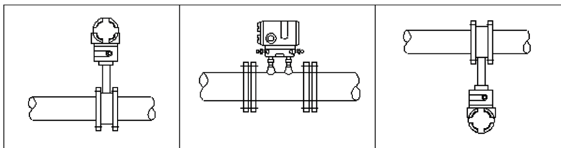
图 9 测气体（对夹式）
