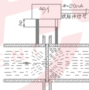
图 2 测量原理示
