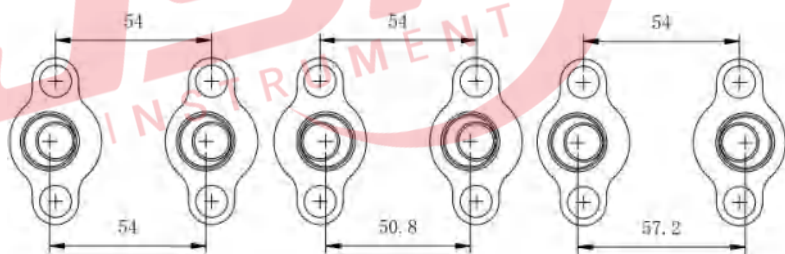
图 2-5 差压变送器连接孔距图
