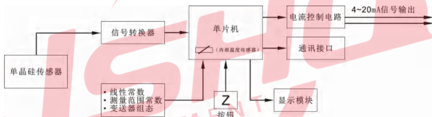
图1-1 变送器原理框图
