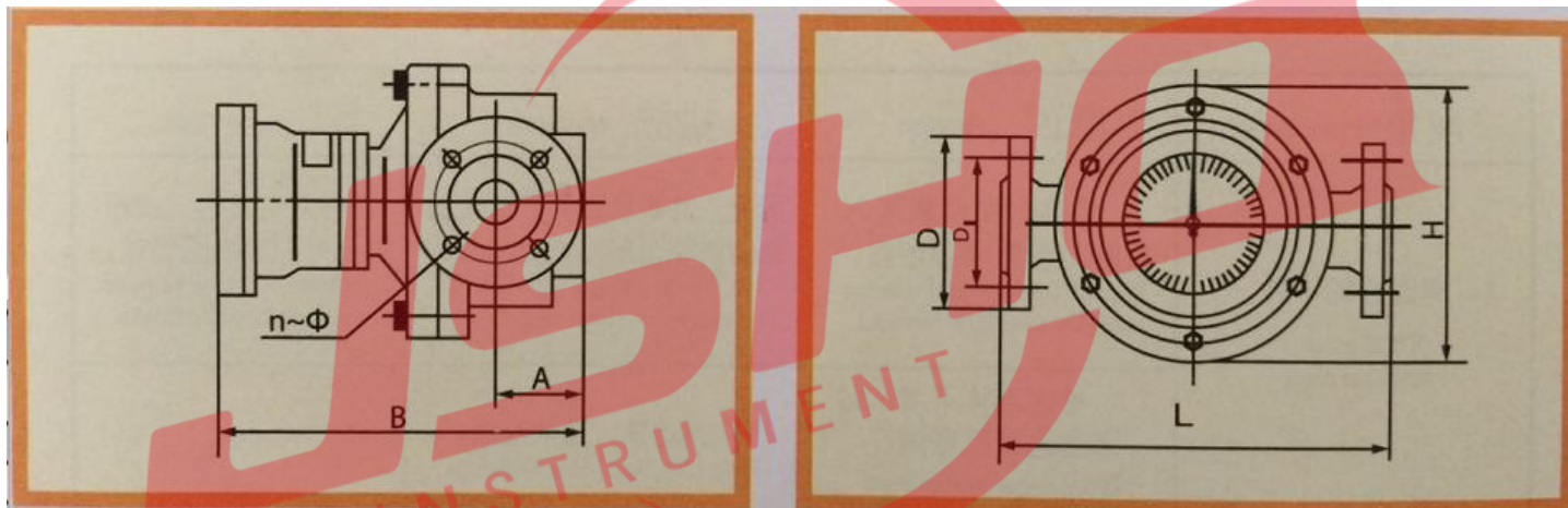
L C- 系列椭圆齿轮流量计外形尺寸 (铸铁、铸钢、不锈钢) LCB- series ellipse gear flowmeter exterior size (cast iron\cast steel\ stainless steel) 单位: mm
